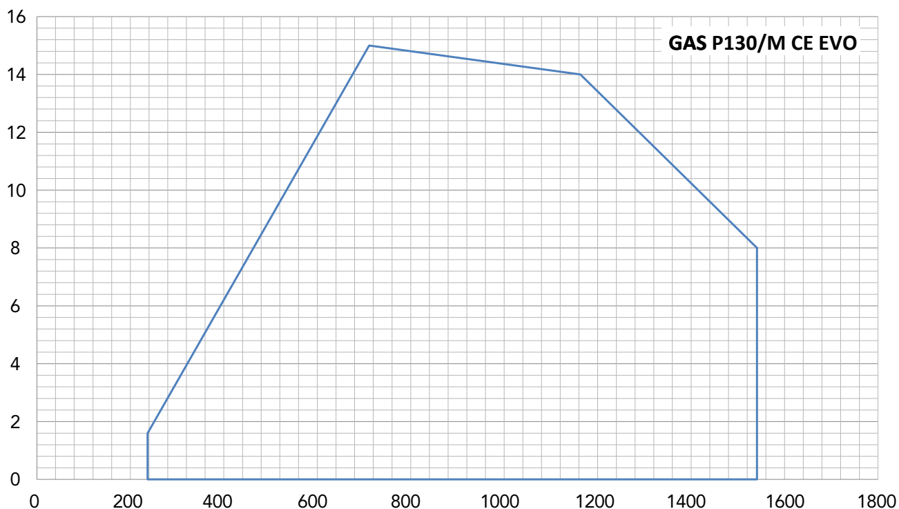
Fig. 2 X = Мощность [кВт] Y = Сопротивление камеры сгорания [мбар]
