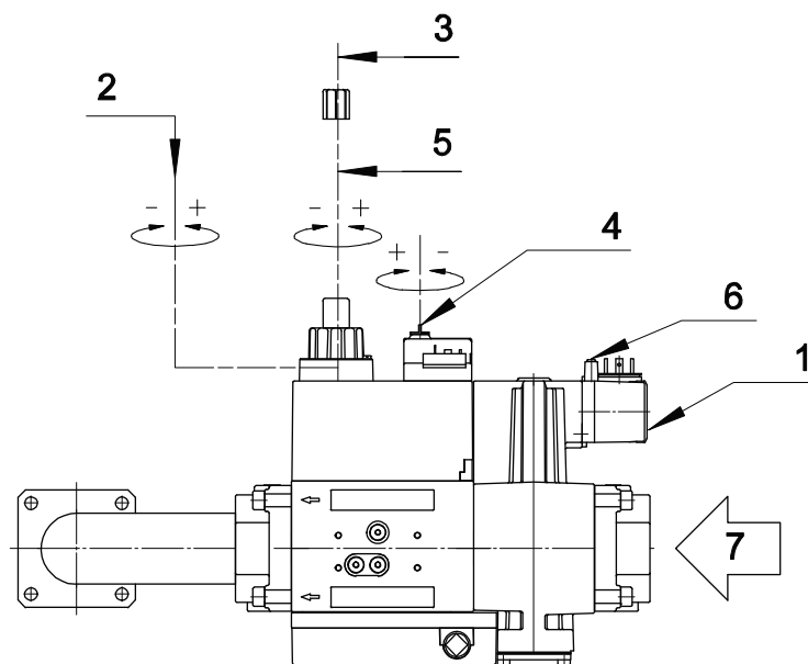
Fig. 16 DUNGS MB-DLE
