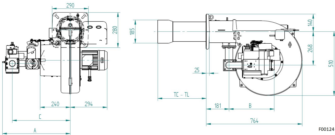
Fig. 5 РАЗМЕРЫ GAS P100/MCE EVO
