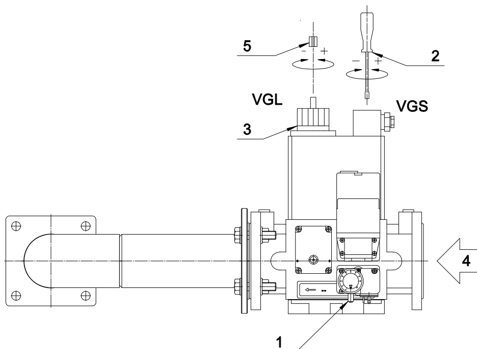
Fig. 17 DUNGS DMV-DLE
