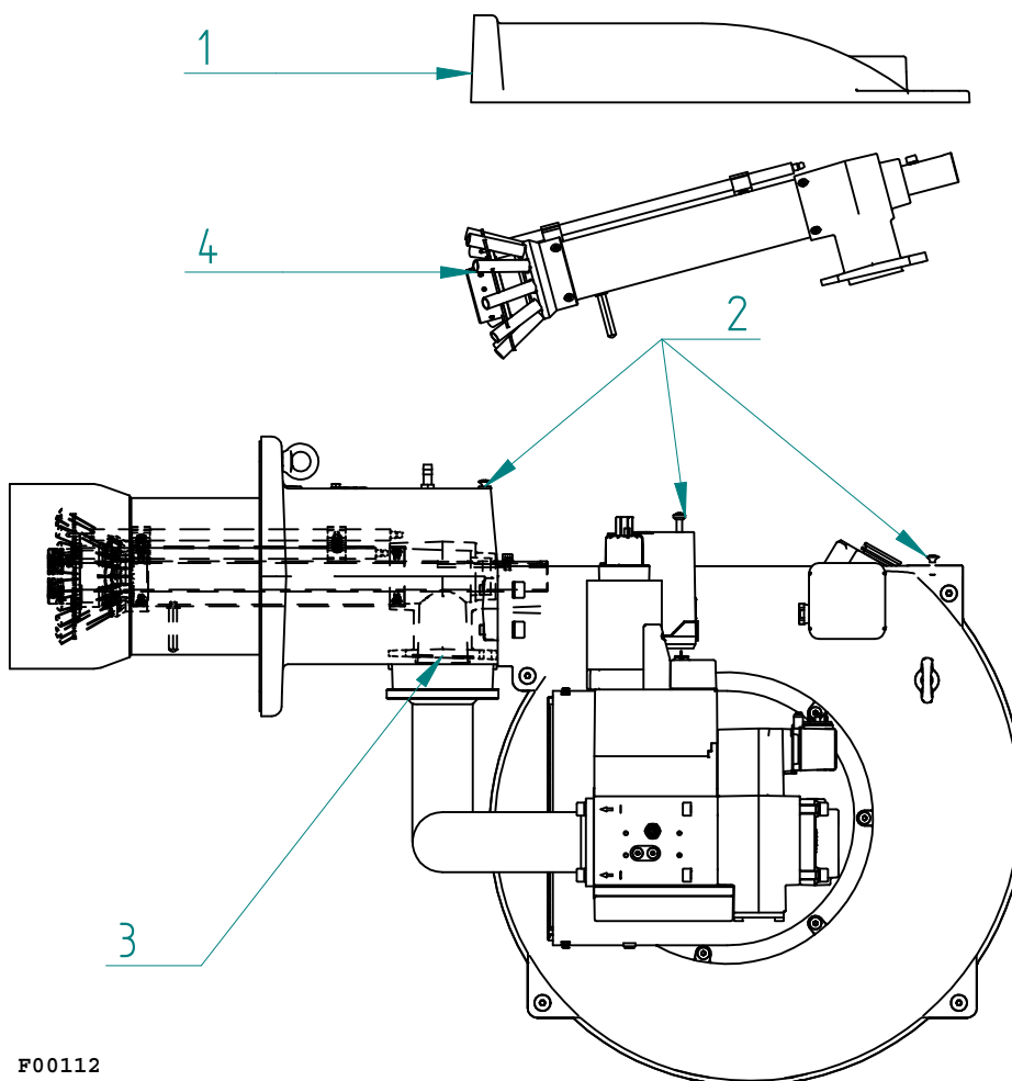
Fig. 19 ИЗВЛЕЧЕНИЕ СМЕСИТЕЛЬНОЙ КАМЕРЫ GAS P100/MCE EVO
